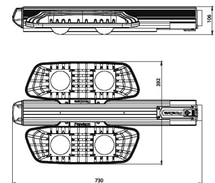
Рисунок 3. Габаритный чертеж
